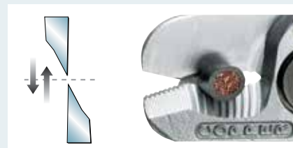
Резка сдвигом
